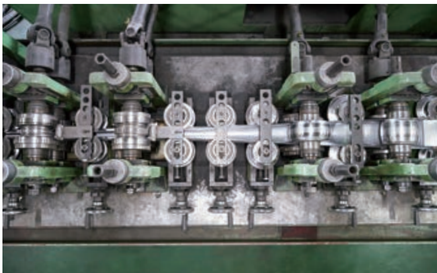
ステンレスパイプの自社製造でコスト削減に貢献する「造管機」
